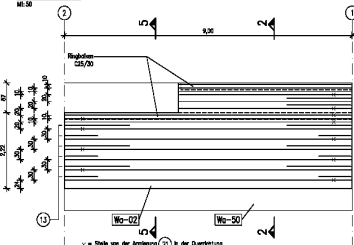
Ansicht West
