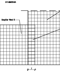
Regeldetail für die Übergreifung der Hauptbewehrung Geogitter
