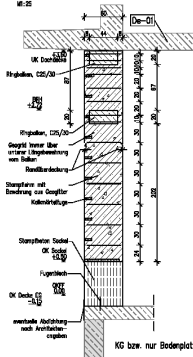
Schnitt 2-2
