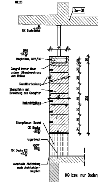
Schnitt 5-5
