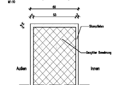
Detail A – Regeldetail Grundriss Wandende mit Bewehrung aus Geogitter
