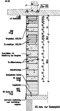
Schnitt 4-4
