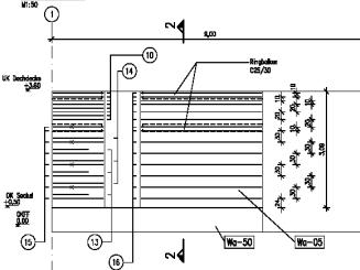
Ansicht Ost
