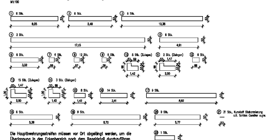
Schneideskizze zur Geogitterbewehrung
