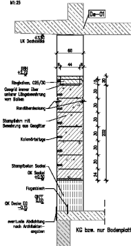
Schnitt 1-1
