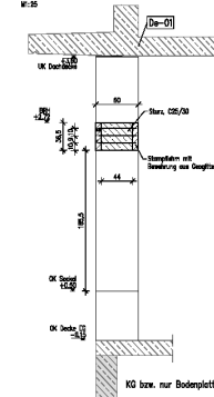
Schnitt 3-3
